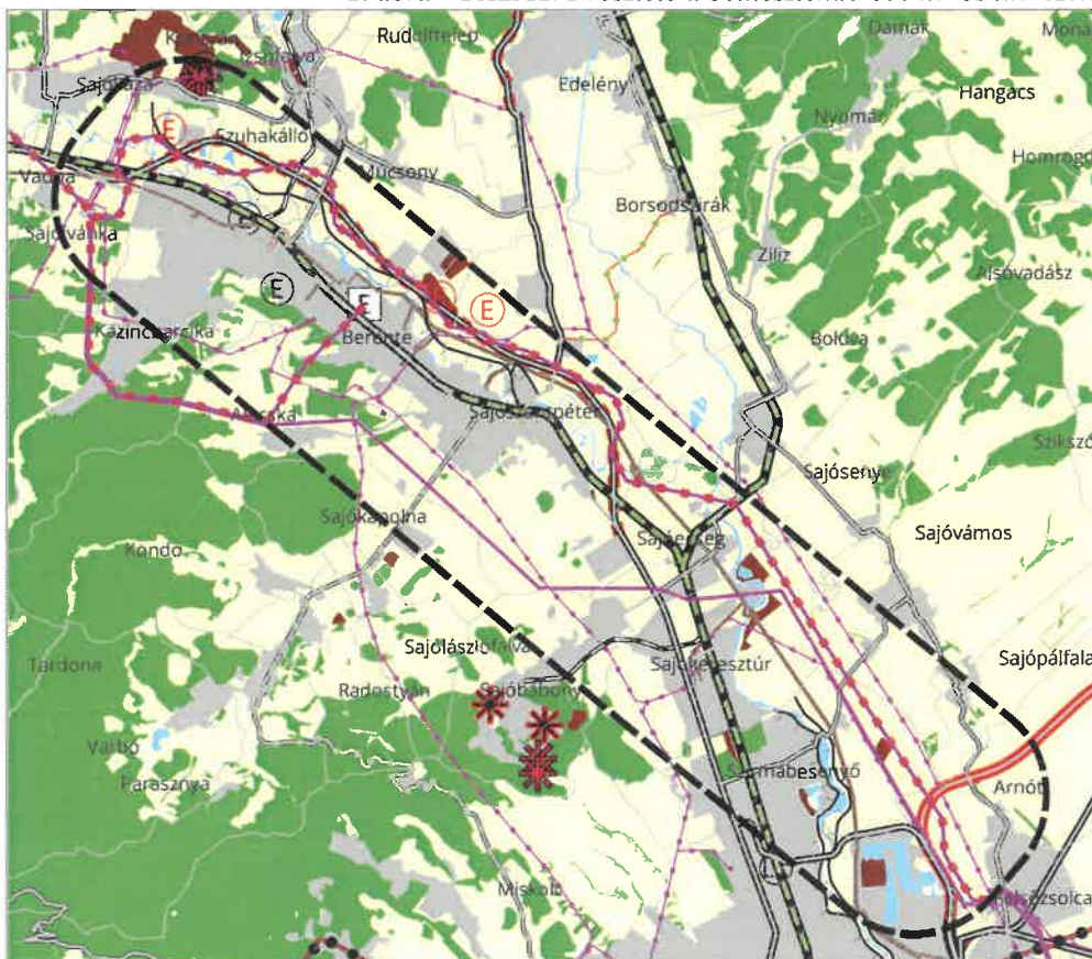
3. ábra – BAZMTrT részlete a beillesztett új 400 KV-os távvezeték nyomvonalával
